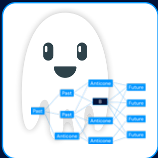
GHOSTDAG Protocol
